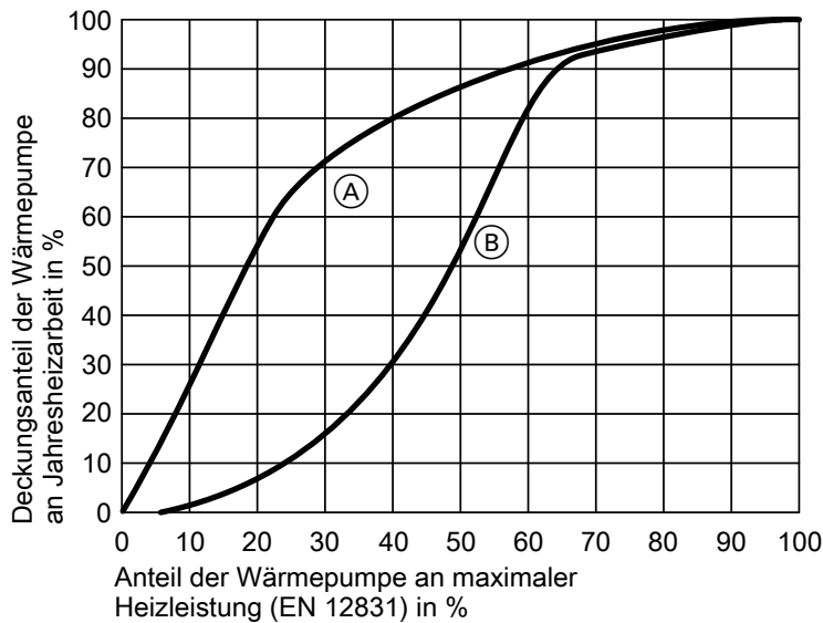
Abb. 16 Deckungsanteil der Wärmepumpe in % an der Jahresheizarbeit (nur Heizbetrieb) eines standardisierten Wohngebäudes, abhängig von der Wärmeleistung der Wärmepumpe und der gewählten bivalenten Betriebsweise
