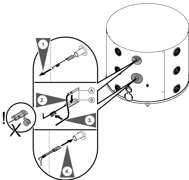
Abb. 7 Beispiel: 75 l
