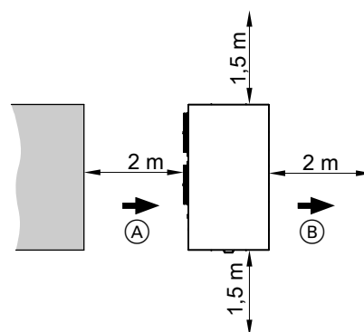
Typ AWO-AC 201.A032 und Typ AWO-AC 202.A064
