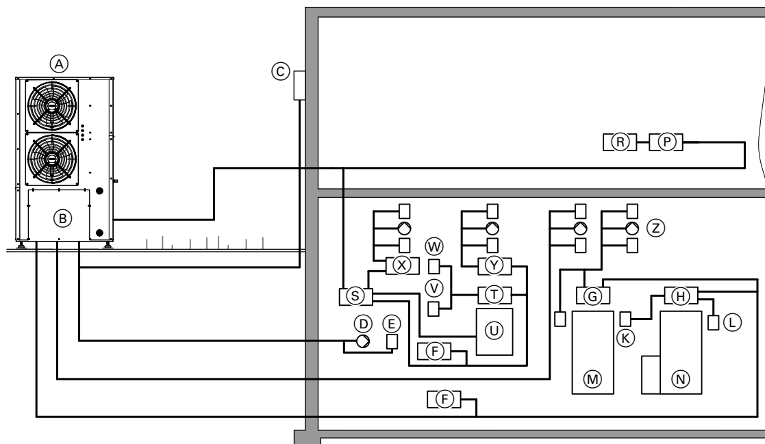
Vitocal 200-A PRO mit Wärmepumpenregler VIRVS und 3 Funktionserweiterungen VIAVS sowie einen weiteren Wärmepumpenregler VIRVS und 3 weitere Funktionserweiterungen VIAVS
