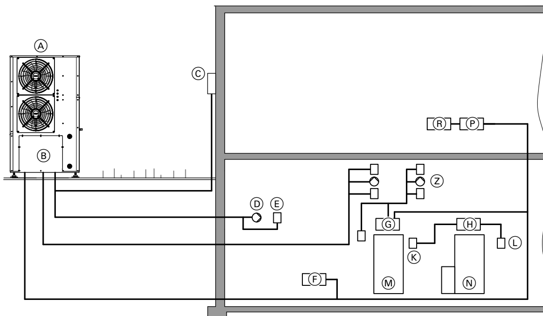
Vitocal 200-A PRO mit Wärmepumpenregler VIRVS und 3 Funktionserweiterungen VIAVS
