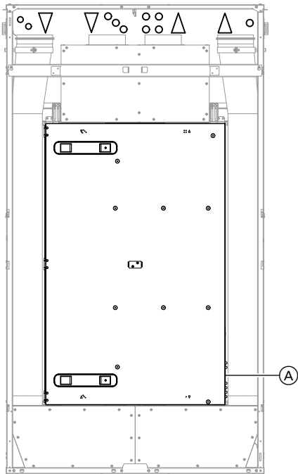
Anschlussvariante 2: Elektrischer Anschlussbereich (A) rechts unten
