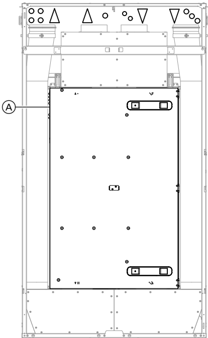
Anschlussvariante 1: Elektrischer Anschlussbereich (A) links oben (Auslieferungszustand)
