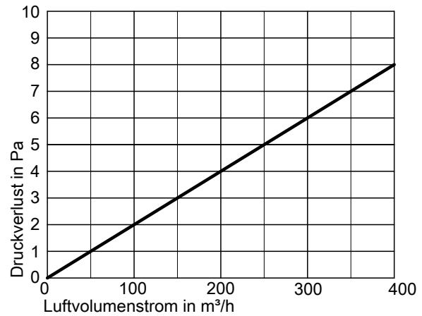
Druckverlust Bogen 90° Kompakt (EPP)
