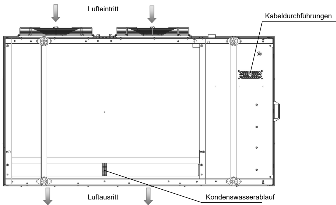
Abb.: Untersicht Typ AWO-AC 202.A064
