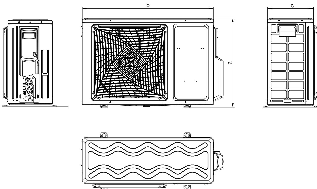
Außeneinheit OFAA200MHA
