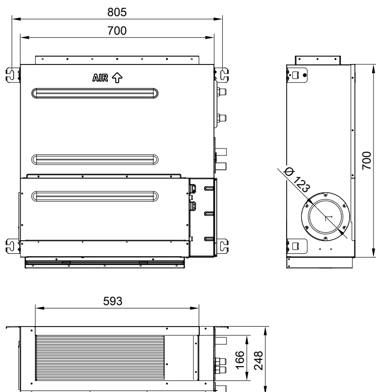
Typ IDMAA200MHA035
