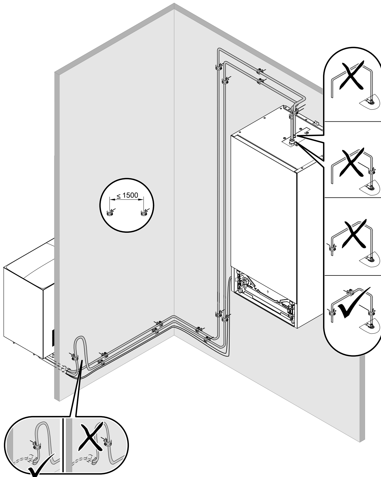
Abb. 21 Rohrbogen in der Heißgasleitung zur Schwingungskompensation innerhalb des Gebäudes
