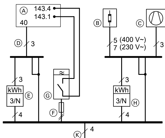
Abb. 50 Darstellung ohne Sicherungen und ohne FI-Schutzschalter
