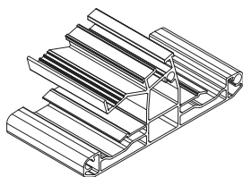
Ⓒ Basisprofil unten
