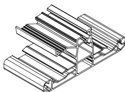
Ⓒ Basisprofil unten
