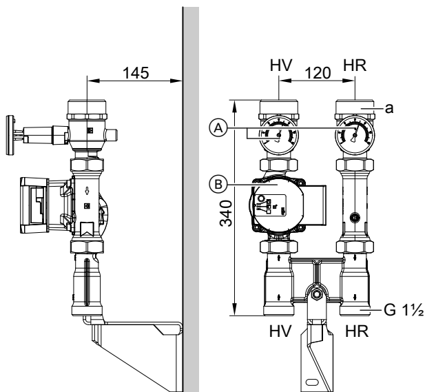
Divicon ohne Mischer: Wandmontage, Darstellung ohne Wärme- dämmung
