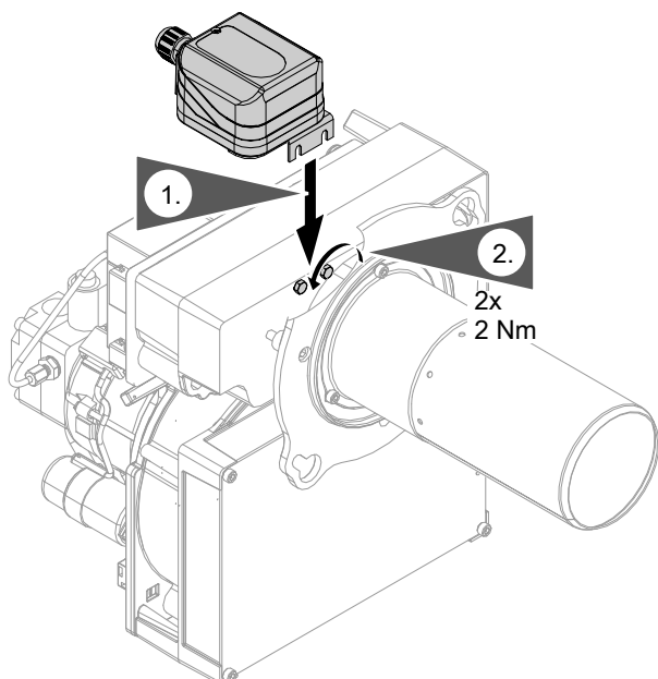
Abb. 1 Ansicht Brenner 18 bis 27 kW
