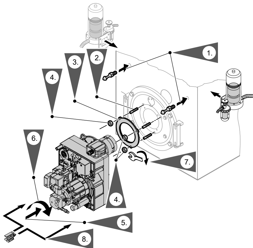
Abb. 5 33 kW Brenner, Ansicht mit Vitoladens 300-T
