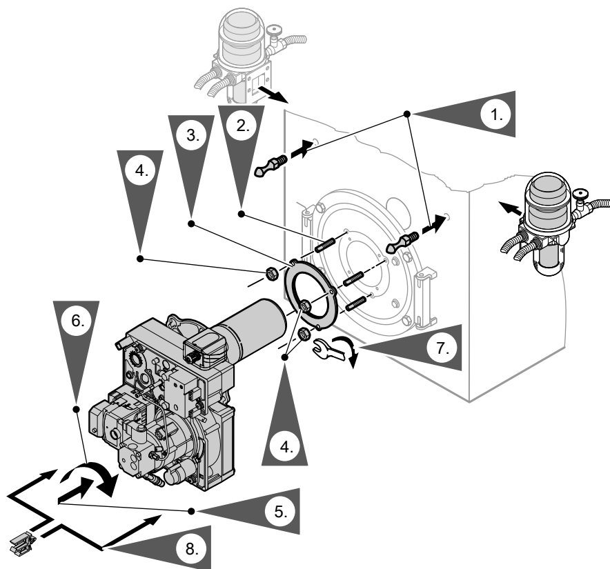
Abb. 4 18 bis 27 kW Brenner, Ansicht mit Vitoladens 300-T
