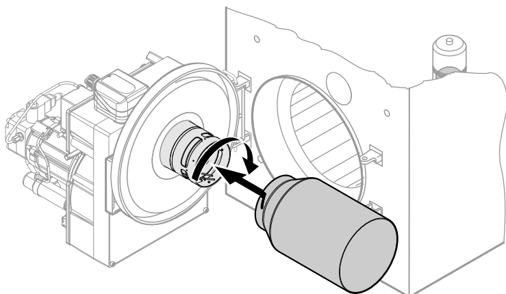
Abb. 6 33 kW Brenner, Flammrohr anbauen
