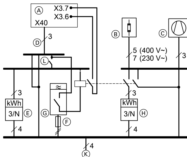
Abb. 50 Darstellung ohne Sicherungen und ohne FI-Schutzschalter
