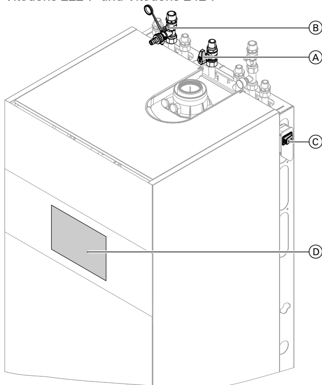
Abb. 15 Beispiel mit Anschlüssen nach oben
