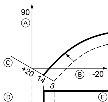
Abb. 66 Beispiel 2: Änderung des reduzierten Raumtemperatur-Sollwerts von 5 °C auf 14 °C
