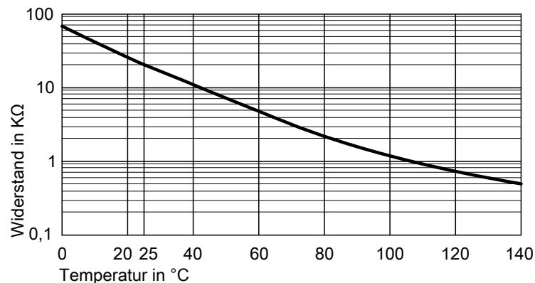
Abb. 60 Sensortyp: NTC 20 kΩ
