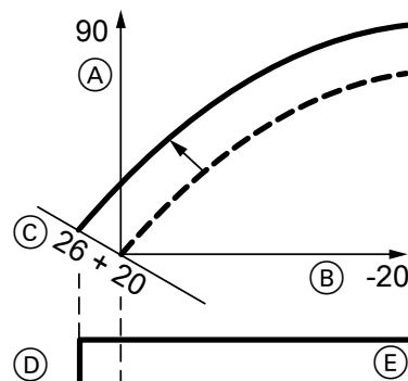
Abb. 65 Beispiel 1: Änderung des Raumtemperatur-Sollwerts von 20 auf 26 °C
