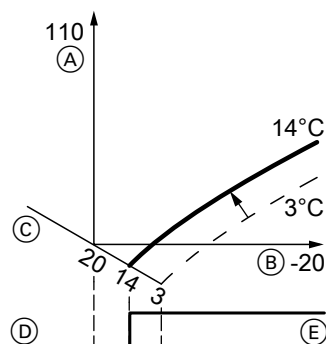
Abb. 37 Änderung des reduzierten Raumtemperatur-Sollwerts von 3 auf 14 °C
