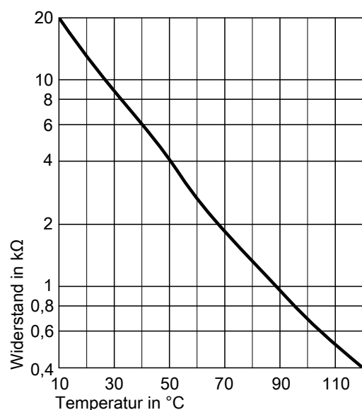
Abb. 48 Sensortyp: NTC 10 kΩ
