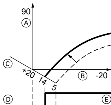
Abb. 37 Beispiel 2: Änderung des reduzierten Raumtemperatur-Sollwerts von 5 °C auf 14 °C
