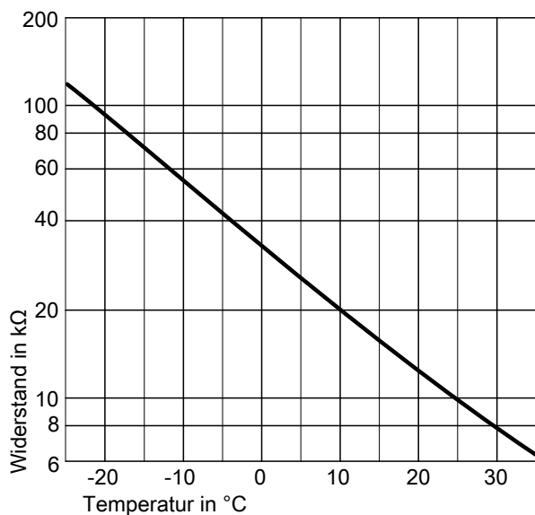
Abb. 46 Sensortyp: NTC 10 kΩ
