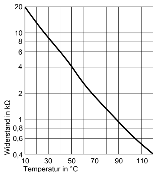
Abb. 50 Sensortyp: NTC 10 kΩ
