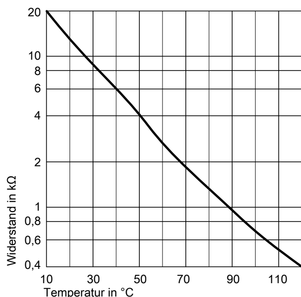
Abb. 53 Sensortyp: NTC 10 kΩ
