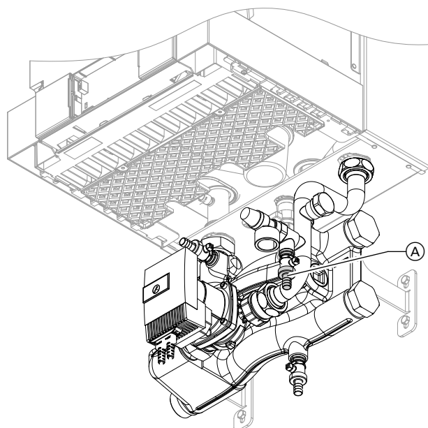
Abb. 20 Anschluss-Set mit integrierter hydraulischer Weiche
