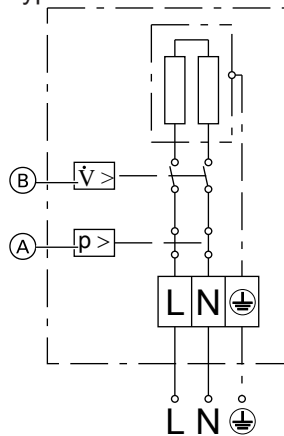
Abb. 10 1/N/PE - 200-240 V
