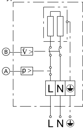
Abb. 11 1/N/PE - 200-240 V
