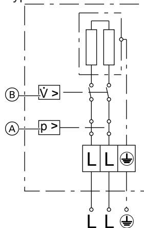
Abb. 12 2/PE - 380-415 V
