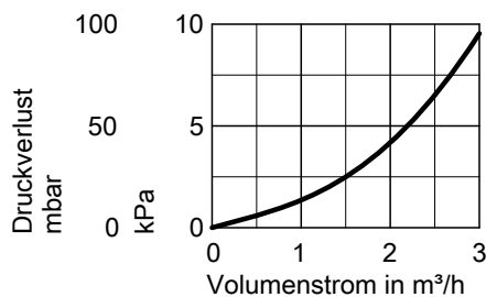
Druckverlustdiagramm
