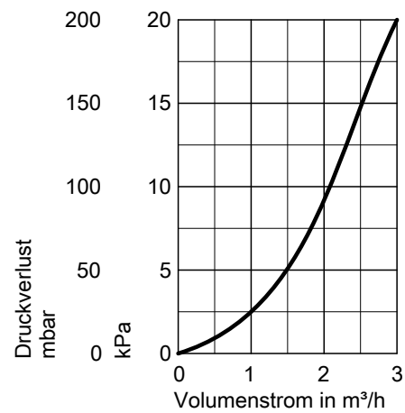
Druckverlustdiagramm
