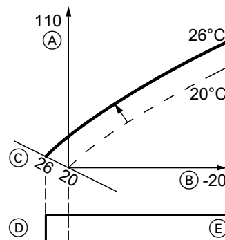
Abb. 21 Änderung des normalen Raumtemperatur-Sollwerts von 20\text{ °C} auf 26\text{ °C}
