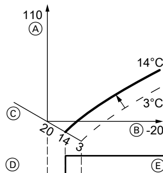
Abb. 22 Änderung des reduzierten Raumtemperatur-Sollwerts von 3 auf 14 °C
