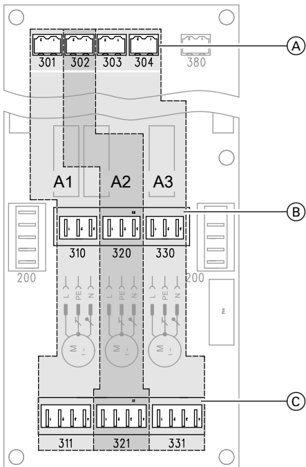
Abb. 18 Leiterplatte HKK
