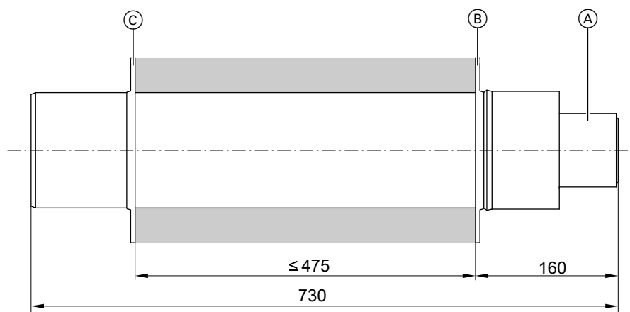
AZ-System Ø 110/150 mm
