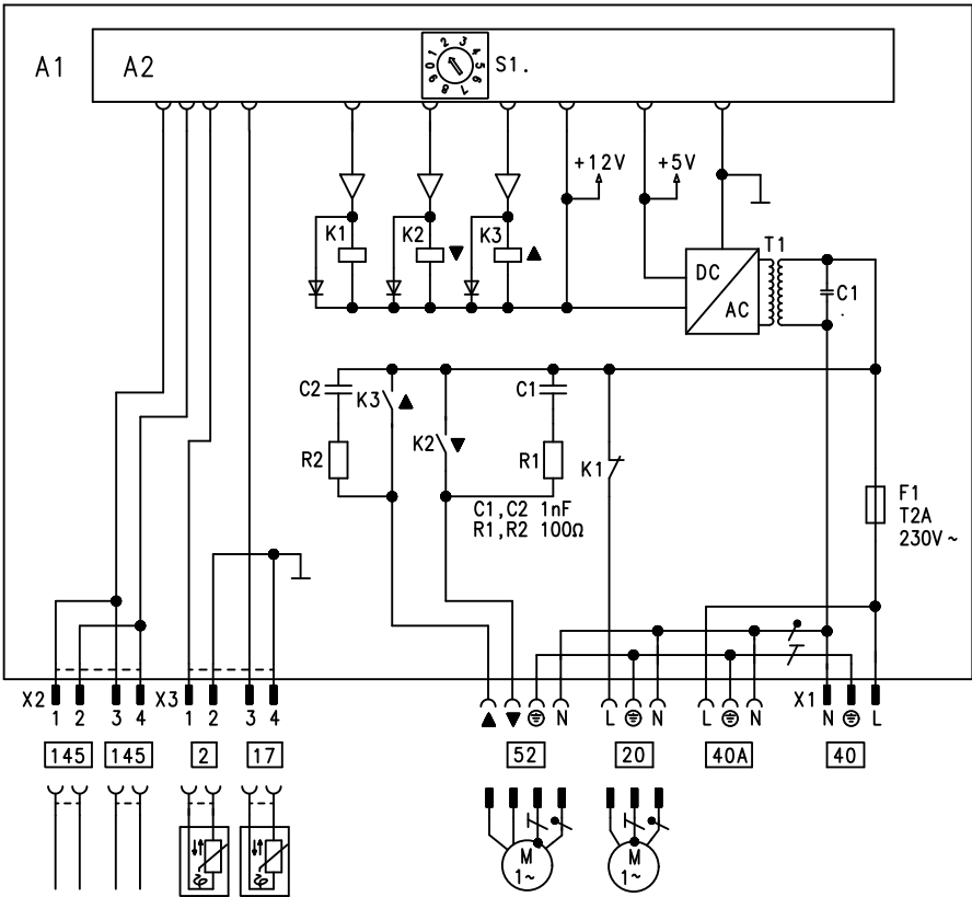
Abb. 53 A1 Grundleiterplatte F1 Sicherung S1 Drehschalter
