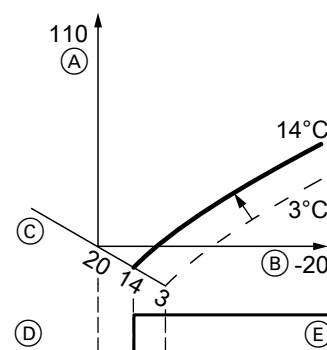
Abb. 27 Änderung des reduzierten Raumtemperatur-Sollwerts von 3\text{ °C} auf 14\text{ °C}
