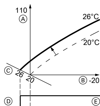
Abb. 26 Änderung des normalen Raumtemperatur-Sollwerts von 20\text{ °C} auf 26\text{ °C}
