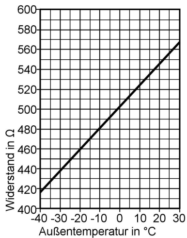
Außentemperatursensor (Ni500)
