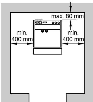
Wandabstände (Draufsicht)
