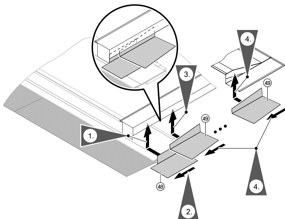
Abb. 35 Aufkantungen der Abdeckhauben flachbiegen.
