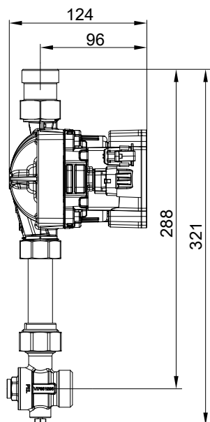
Abmessungen Zirkulations-Set für Typ PBSA, PZSA
