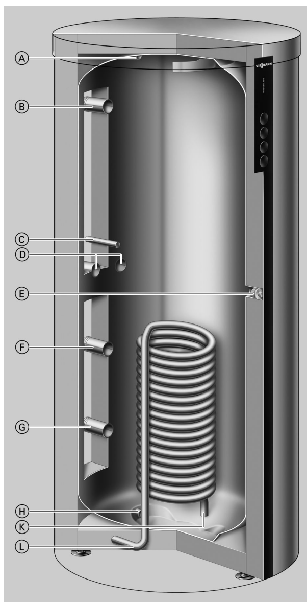
Vitocell 140-E (Typ SEIA) – Multivalenter Heizwasser-Pufferspeicher
