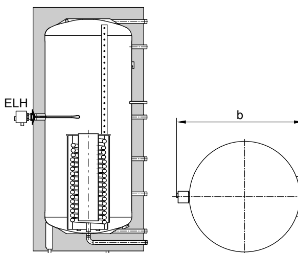
Vitocell 160-E mit Elektroheizeinsatz EHE
