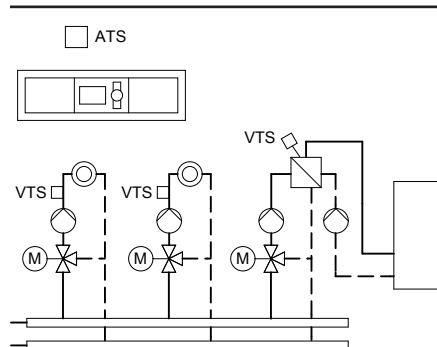
Speicherladesystem mit Mischgruppe
