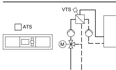
Speicherladesystem mit Mischgruppe
