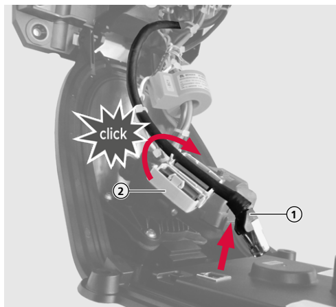
Fig. 5: Sette på klemferritten
