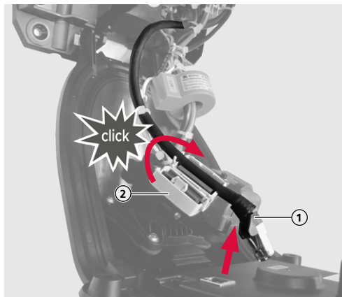
Fig. 5: Applicare la ferrite pieghevole
