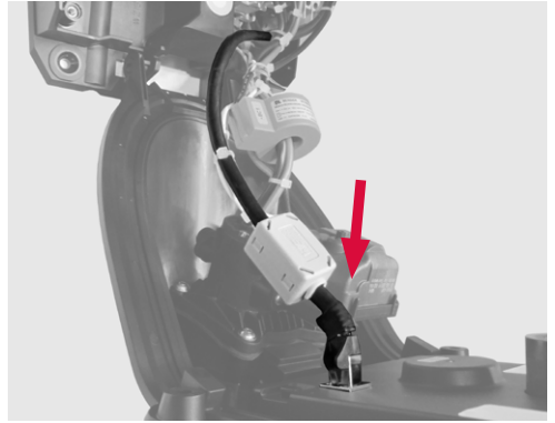
Afb. 6: Leiding insteken
