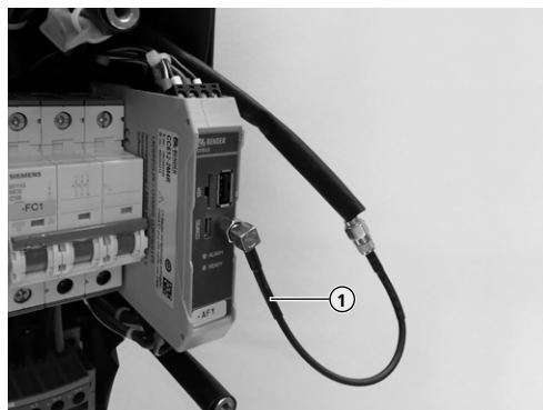
Fig. 3: montage de la rallonge d'antenne
