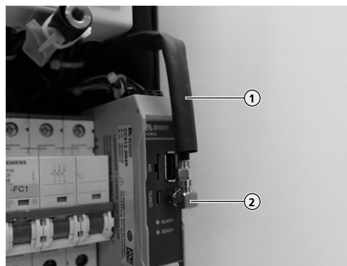
Fig. 2: Allentare l'antenna e l'adattatore angolare
