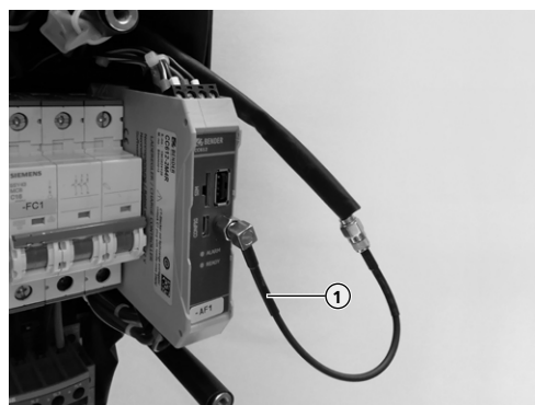
Fig. 3: Montaggio della prolunga antenna
