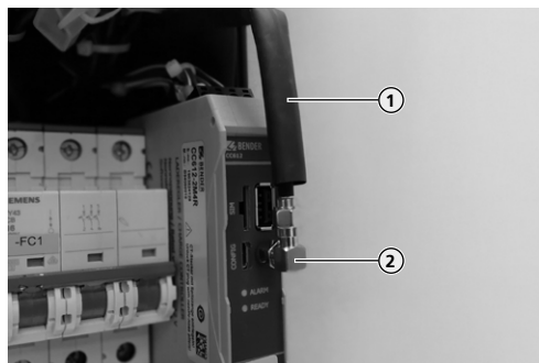
Fig. 2: Débranchement de l'antenne et de l'adaptateur coudé
