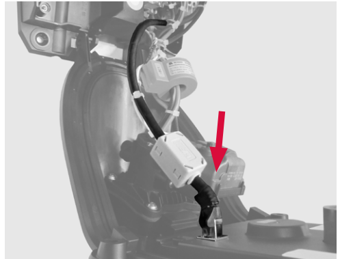
Fig. 6: Branchement du câble
