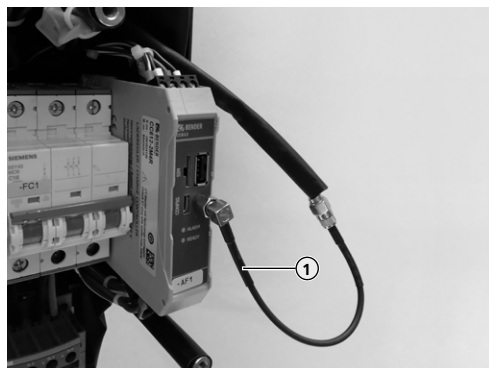
Fig. 3: Montaje de la prolongación de antena
