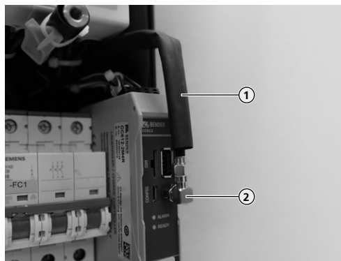
Fig. 2: Retirada de la antena y del adaptador de ángulos
