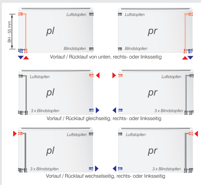
Abbildung 3: Anschlussvarianten Wärmepumpenheizkörper PLAN
