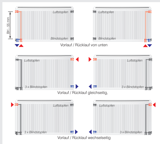
Abbildung 4: Anschlussvarianten Wärmepumpenheizkörper UNIVERSAL
