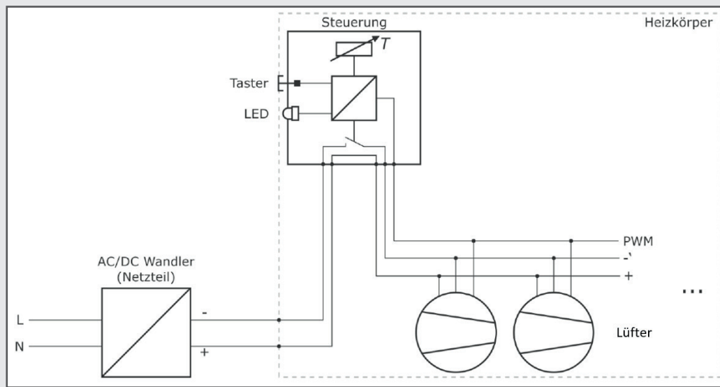
Abbildung 17: Schematisches Schaltbild
