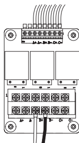
4. Kurzschlusskabel entfernen
