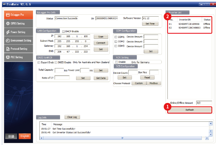
Abbildung 5.2-12 Abruf des Wechselrichterstatus
