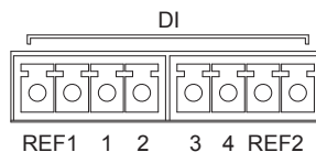
Abbildung 4.5-1 Schema des DI-Anschlusses des EzLoggers Pro
