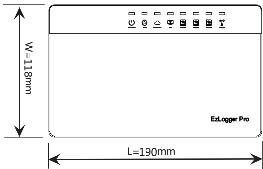
Abbildung 2.2-2 Vorderansicht des Gehäuses des EzLoggers Pro
