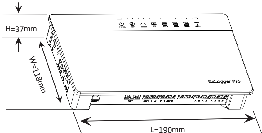
Abbildung 2.2-1 Außenansicht des EzLoggers Pro
