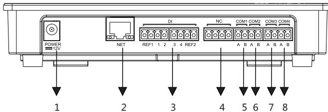
Abbildung 4.1-1 Schema der Anschlüsse des EzLoggers Pro auf der Unterseite
