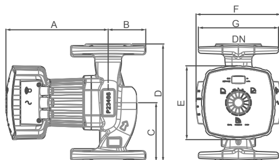
Abb. 3: Pumpenaggregat mit Flansanschluss
