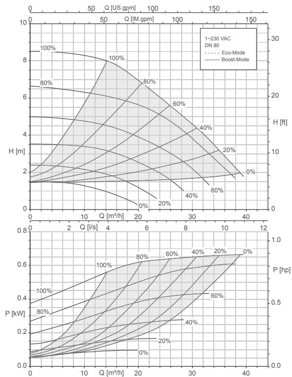
Calio 80-80 Stellerbetrieb, Eco-Mode
