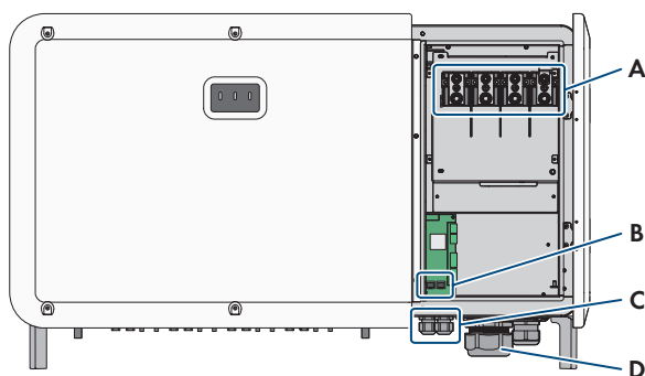
Abbildung 7: Anschlussbereiche im Inneren des Wechselrichters
