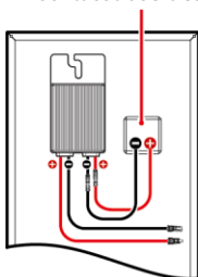
Anschlussdose des PV-Moduls
