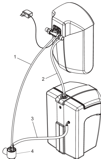
Abb. 12: Anschluss an Siphon
