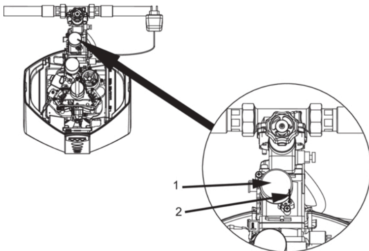
Abb. 14: Leckageschutz-System
