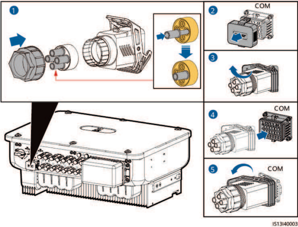
Abbildung 5-13 Sichern des Signalkabelanschlusses
