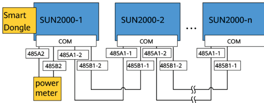
Abbildung 5-14 Smart Dongle-Netzwerkaufbau
