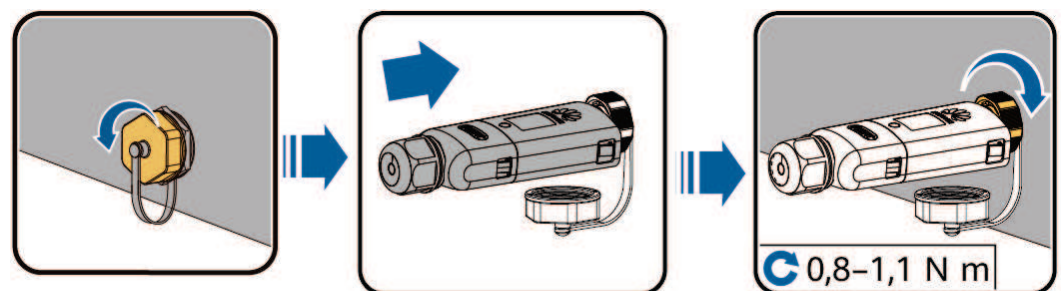
Abbildung 5-10 Anschließen eines WLAN-FE Smart Dongle (WLAN-Kommunikation)
