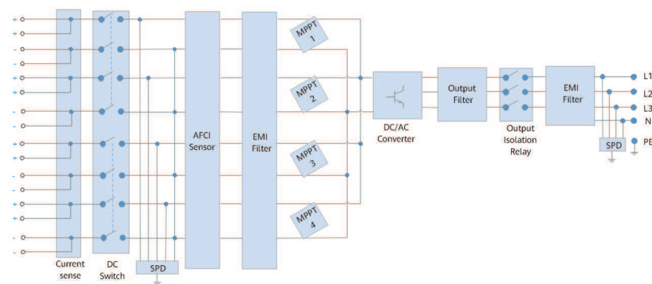
Abbildung 2-6 Schaltplan
