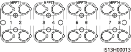
Abbildung 5-7 DC-Eingangsklemmen
