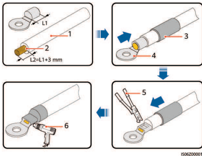
Abbildung 5-2 Crimpen eines Kabelschuhs
