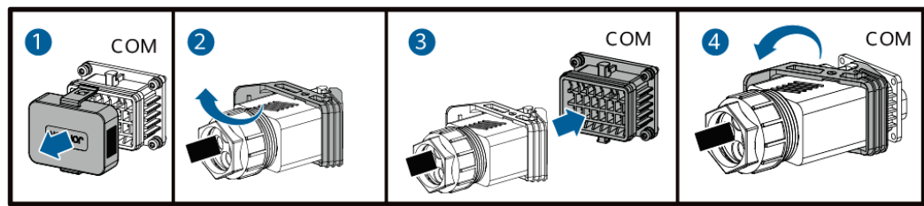
Abbildung 5-24 Sichern des Signalkabelanschlusses
