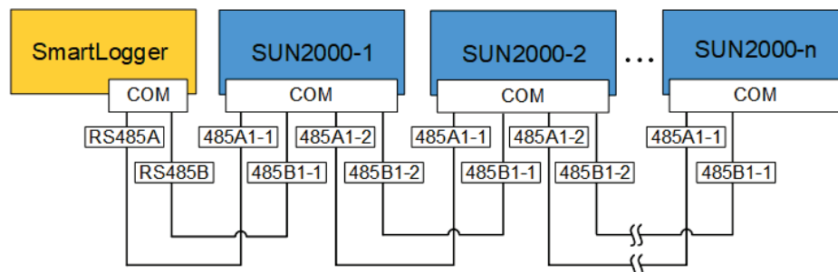
Abbildung 5-15 SmartLogger-Netzwerkaufbau
