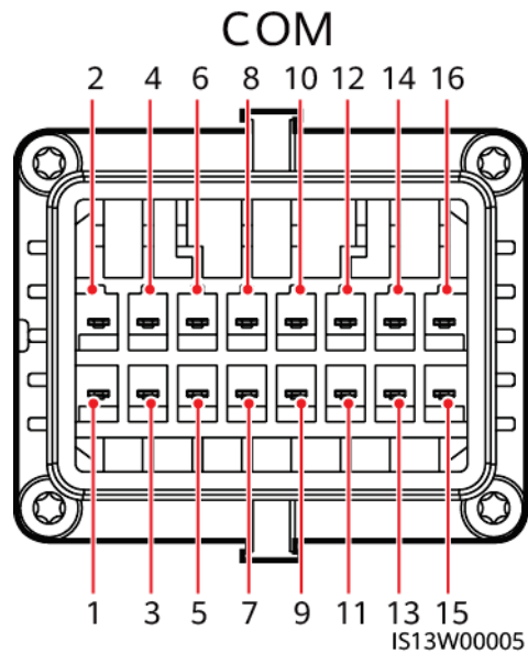
Abbildung 5-12 Definition der Pins
