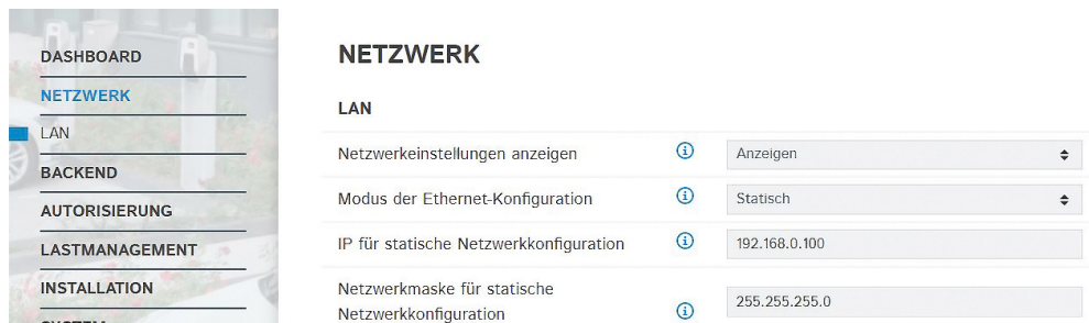
Abb. 11: Weboberfläche von allen vernetzten Ladestationen zur Konfiguration von statischen IP-Adressen
