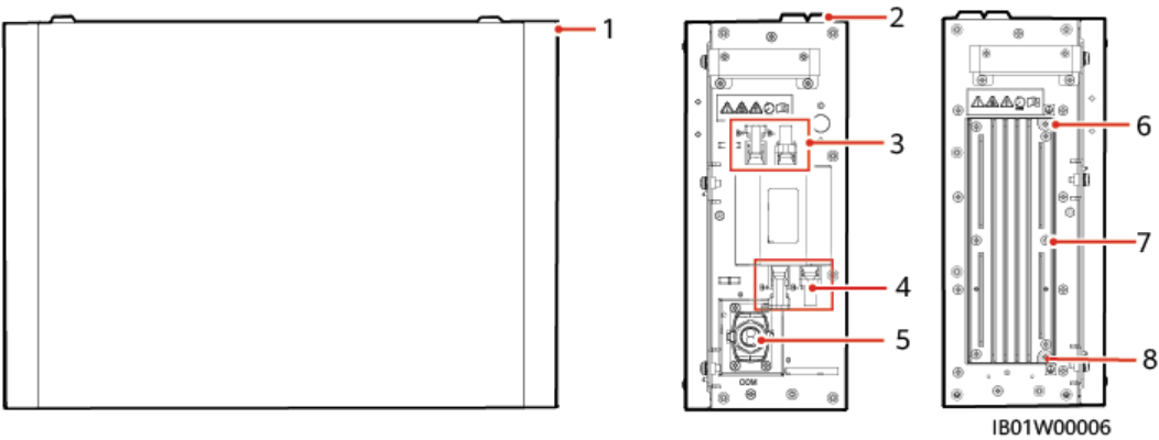
Abbildung 2-8 Akkuerweiterungsmodul
