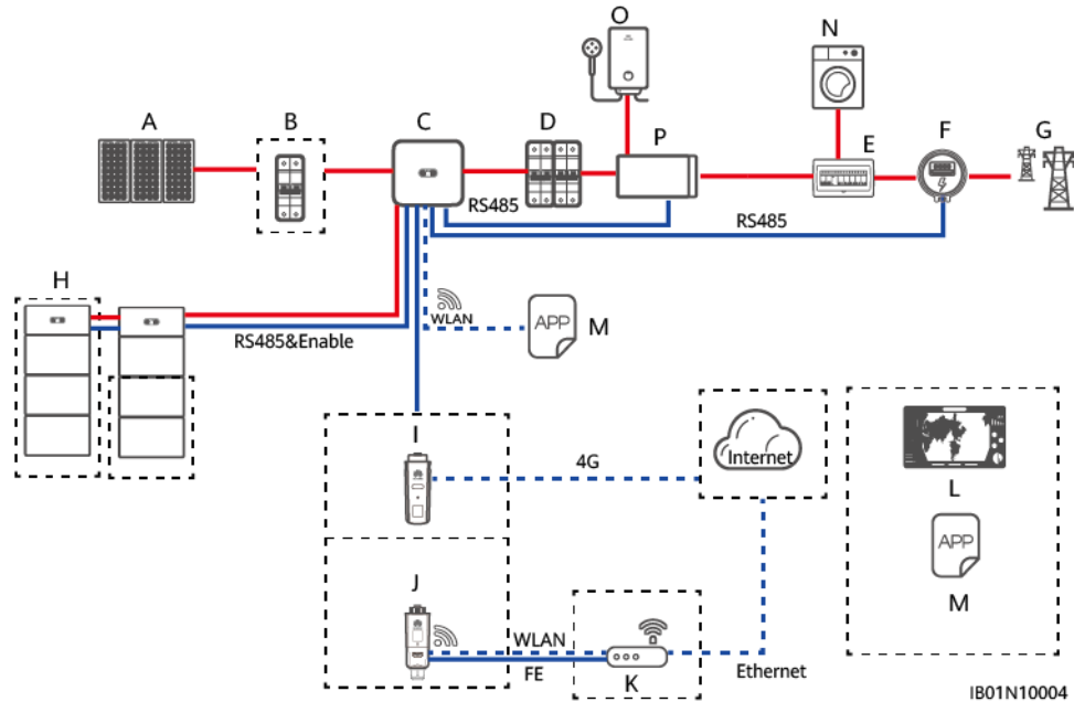
Abbildung 3-9 Grundlegende Vernetzung des parallelen netzentkoppelten ESS (Gestrichelte Kästchen stehen für optionale Komponenten.)
