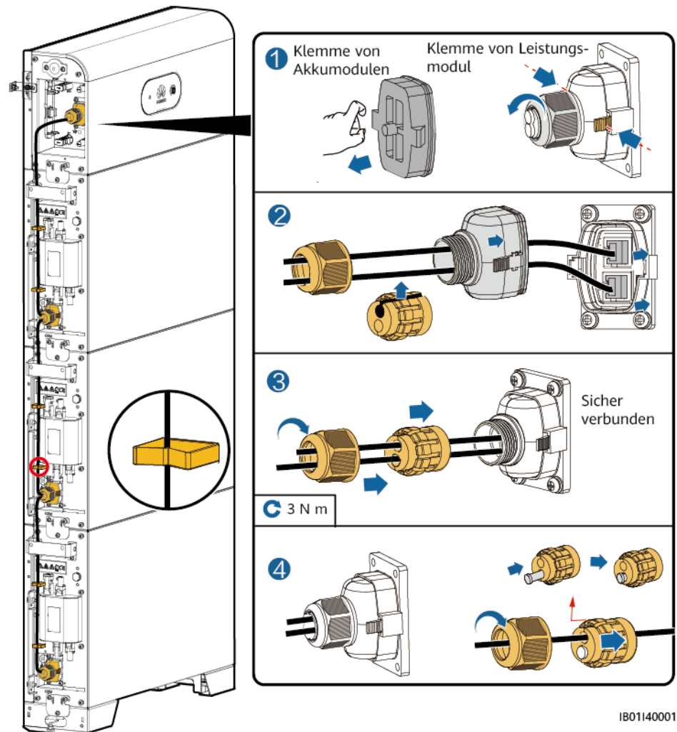
Abbildung 5-4 Signalkabelverbindungen zwischen dem Leistungssteuermodule und den Akkuerweiterungsmodulen
