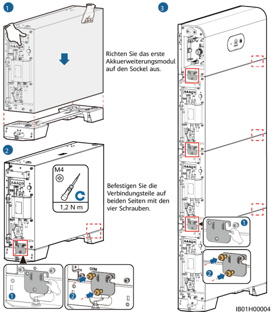
Abbildung 4-5 Installieren der Akkuerweiterungsmodule und des Leistungssteuermoduls
