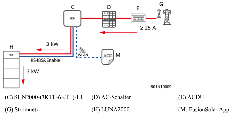
Abbildung 7-2 Netzwerkdiagramm für Szenario mit einphasiger Stromversorgung
