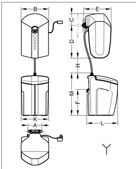
Abb. 20: Einbaumaße
