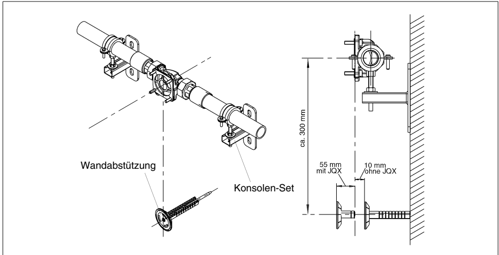
Abb. 5: Wandabstützungskomponenten
