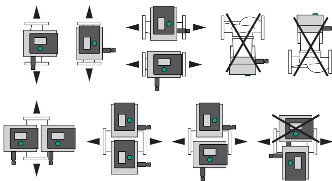
Fig. 10: Zulässige Einbaulagen
