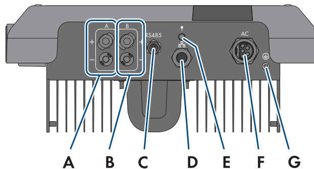
Abbildung 6: Anschlussbereiche an der Unterseite des Wechselrichters
