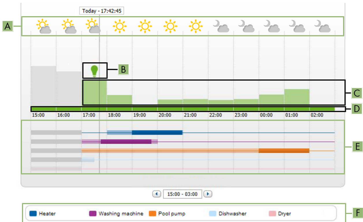
Abbildung 8: Diagramm Prognose und Handlungsempfehlung (Beispiel)
