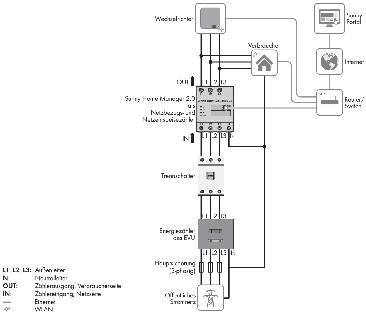
Abbildung 4: Anschlussbeispiel in TN- und TT-Stromnetzen bei Installation am Netzanschlusspunkt unter Verwendung der integrierten Messeinrichtung
