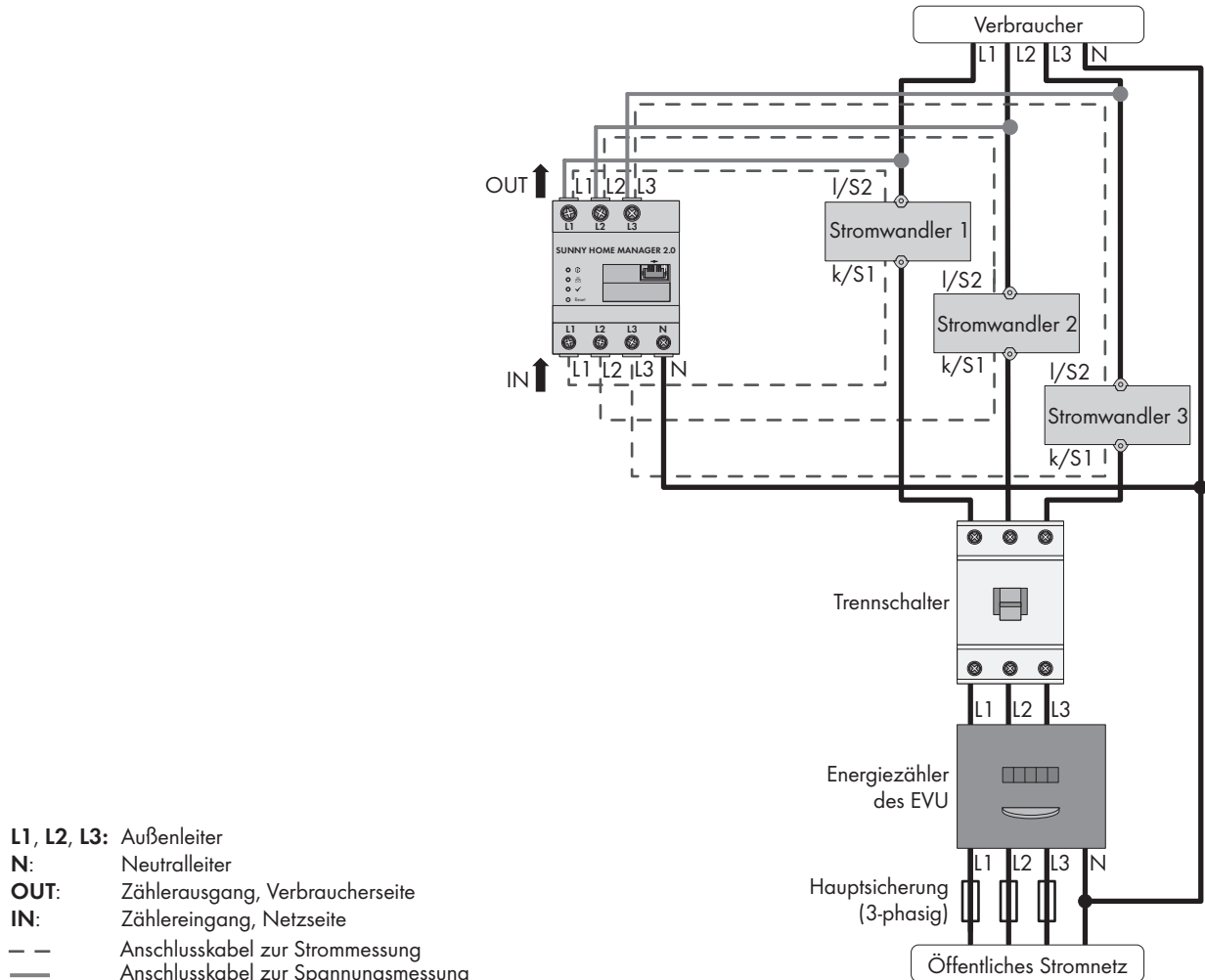
Abbildung 5: Anschlussbeispiel in TN- und TT-Stromnetzen bei Installation am Netzanschlusspunkt
