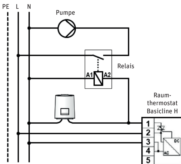
Anschluss mit Raumthermostat Basicline H
