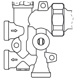
Im Betrieb: Absperrventil wieder öffnen!
