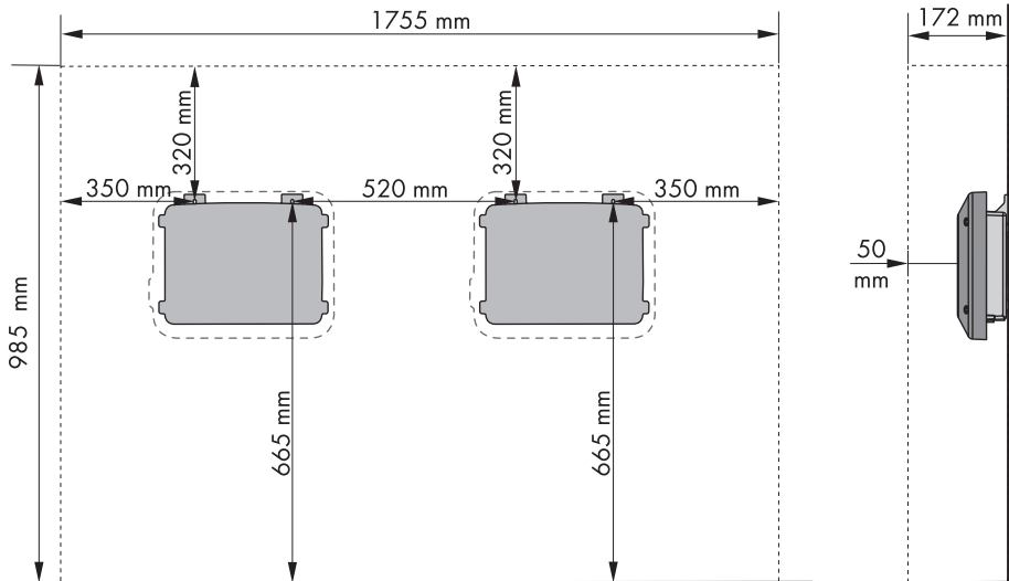
Abbildung 4: Empfohlene Abstände
