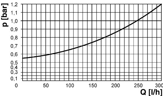
Bild 1: Rücklaufdruck
