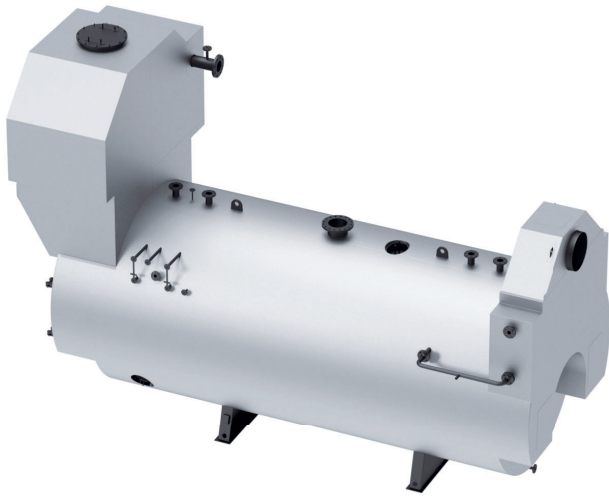
Dampfkessel mit Überhitzer- modul für erhöhte Dampf- anforderungen
