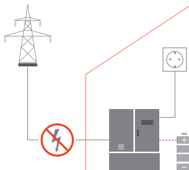
Schwarzstart PRO – damit lassen sich Vitobloc Blockheizkraftwerke bei einem Netzausfall ohne externe Energiezufuhr starten.
