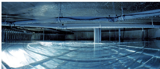
Blick in das Innere des Eis-Energiespeichers – hier im vereisten Zustand.
