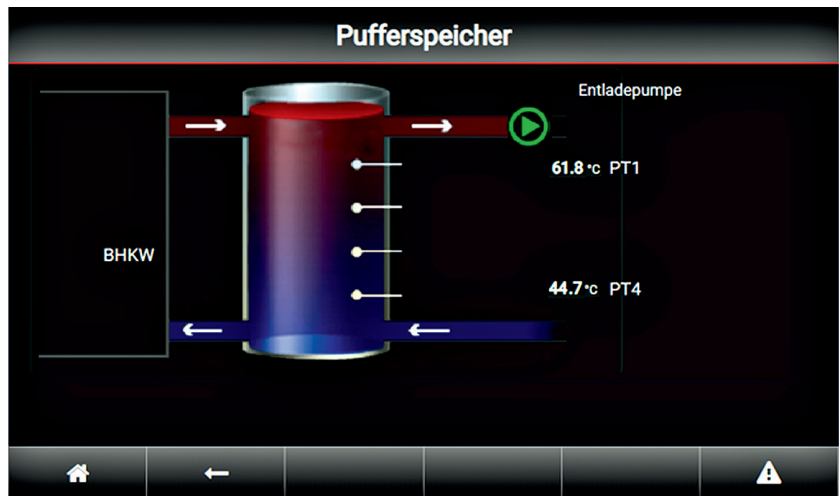
ViNCI Buffer-Management (BM) Übersichtliche Darstellung auf dem Display des Vitobloc 200 NG 260.
