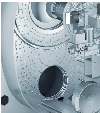
Korrosionsbeständige Inox-Crossal-Wärmetauscherfläche aus Edelstahl Rostfrei für hohe Betriebssicherheit und lange Nutzungsdauer
