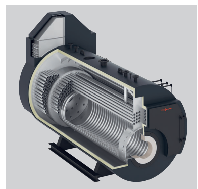
Befuerter Dreizugkessel zur Hochdruck-Dampferzeugung mit integriertem Economiser
