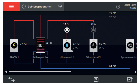
Übersichtlich gestaltetes Anlagenschema mit Anzeige der relevanten Anlagendaten und direktem Zugriff auf Wärmeerzeuger, Warmwasserspeicher und Verbraucher sowie Zugang zu der Störmeldezentrale und den Trenddaten.
