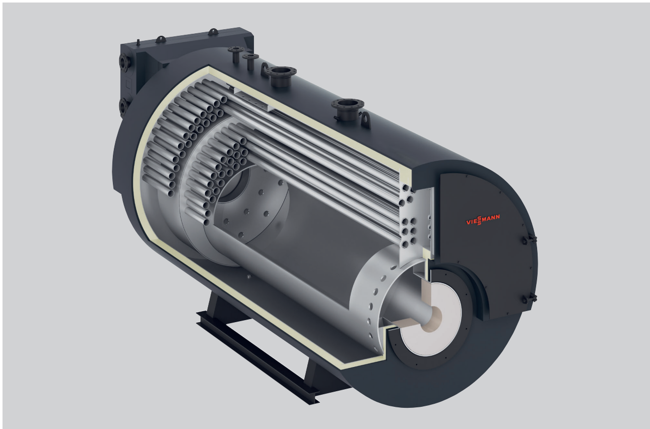
Befuerter Dreizugkessel zur Niederdruck-Heißwassererzeugung mit integriertem Brennwert-Wärmetauscher
