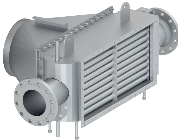
Integrierter Abgas-/Wasser-Wärmetauscher
